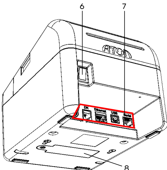
Рисунок 2. Вид снизу/сзади/слева
